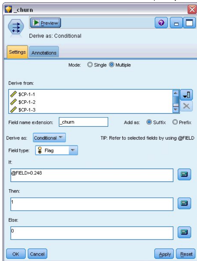
Figura 375. Nodo Derivar: pestaña Configuración
