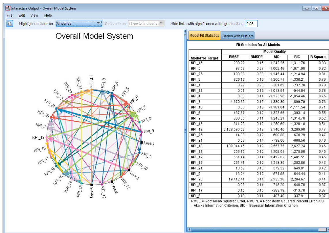
Figura 401. Sistema de modelo global, vista para todas las series
