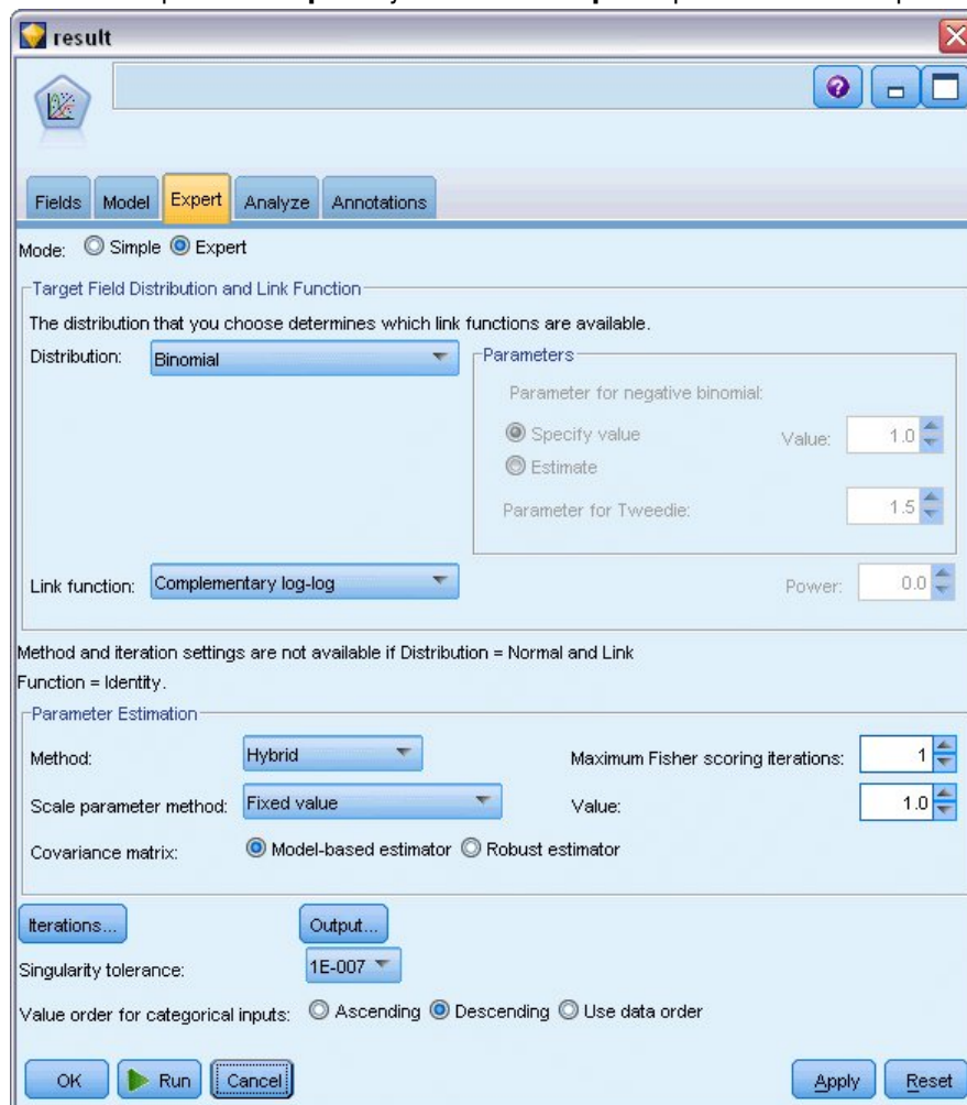
Figura 300. Selección de opciones de experto
