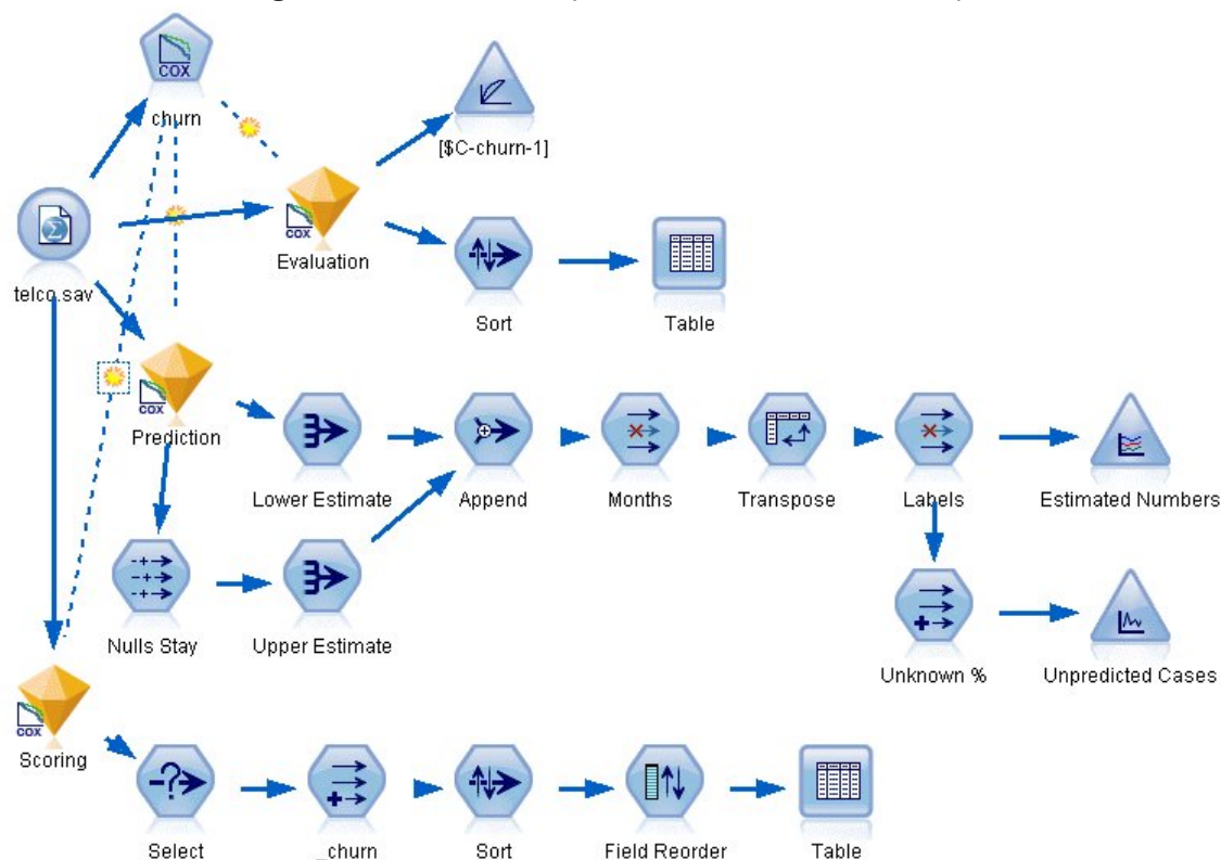
Figura 339. Ruta de ejemplo para analizar el tiempo de abandono
