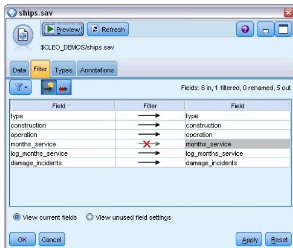
Figura 311. Filtrado de un campo innecesario
