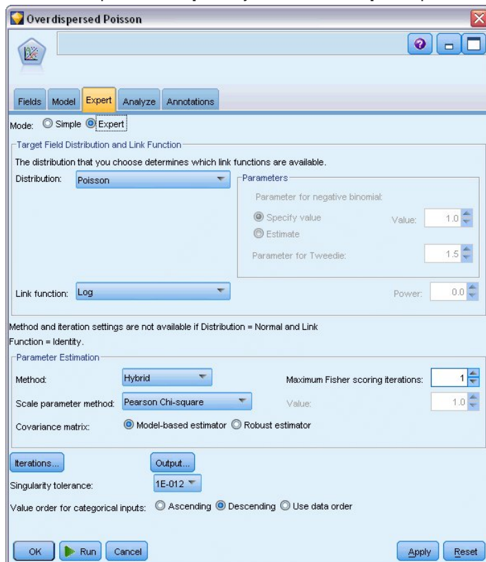
Figura 314. Selección de opciones de experto
