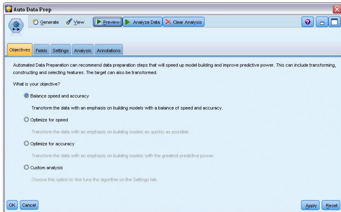
Figura 53. Objetivos ADP predeterminados
