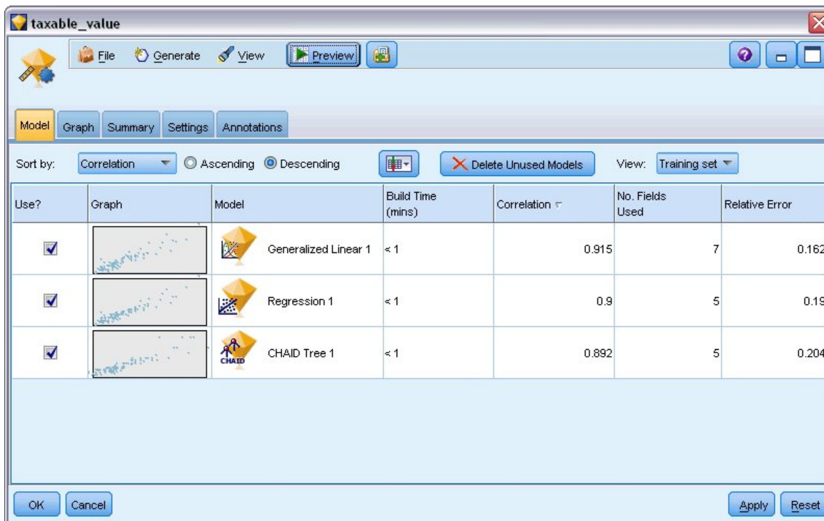
Figura 48. Resultados Autonuméricos
