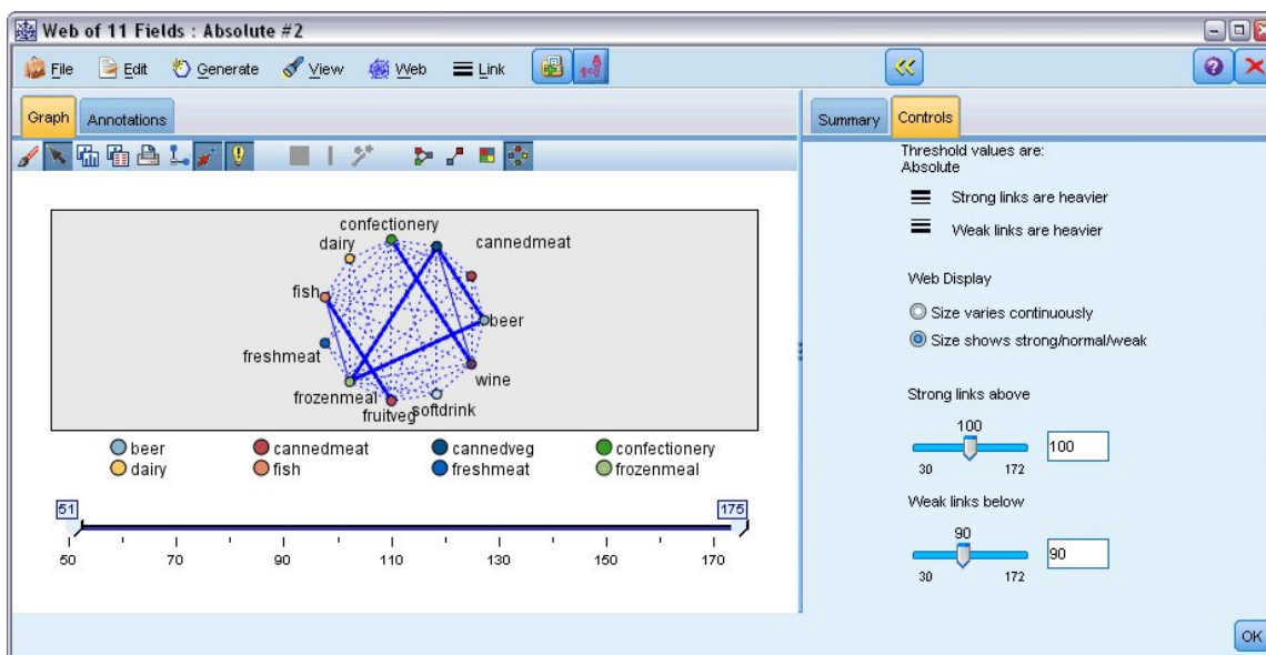
Figura 384. Visualización de malla restringida
