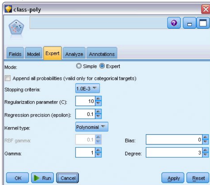
Figura 336. Configuración de la pestaña Experto para Polinómica
