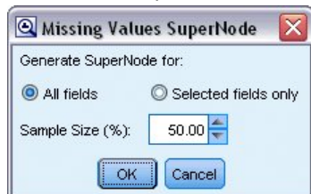
Figura 162. Especificación del tamaño de la muestra
