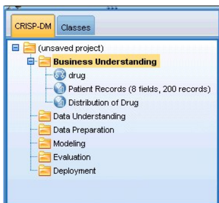
Figura 8. Vista CRISP-DM
