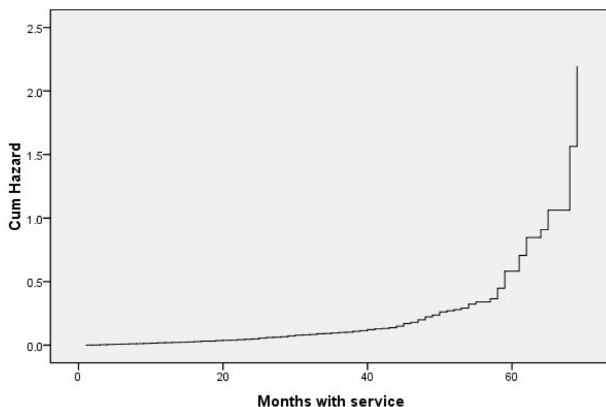
Figura 352. Curva de riesgo de cliente "promedio"
