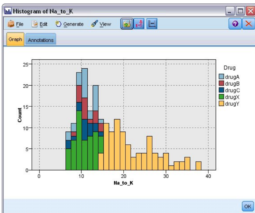
Figura 92. Visualización del histograma
