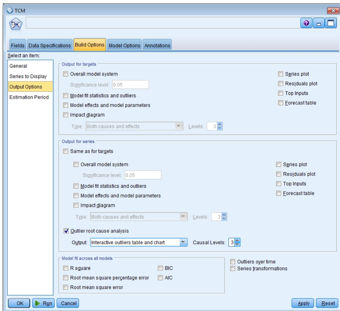
Figura 407. Opciones de salida de modelo causal temporal
