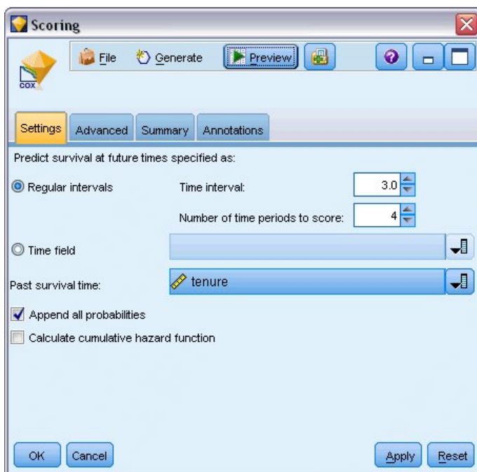
Figura 373. Nugget de Coxreg: pestaña Configuración
