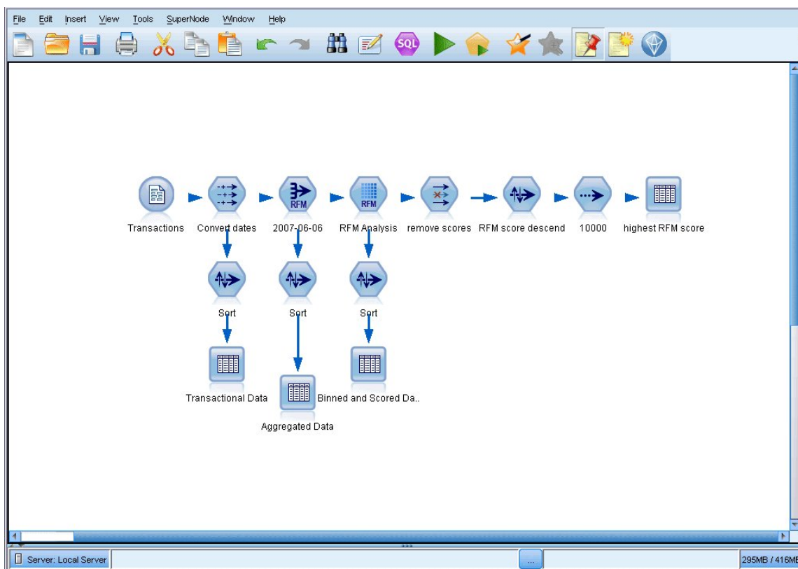
Figura 10. Lienzo de rutas maximizado
