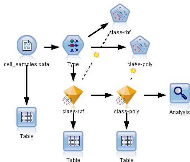
Figura 327. Ruta de ejemplo para el modelado de SVM
