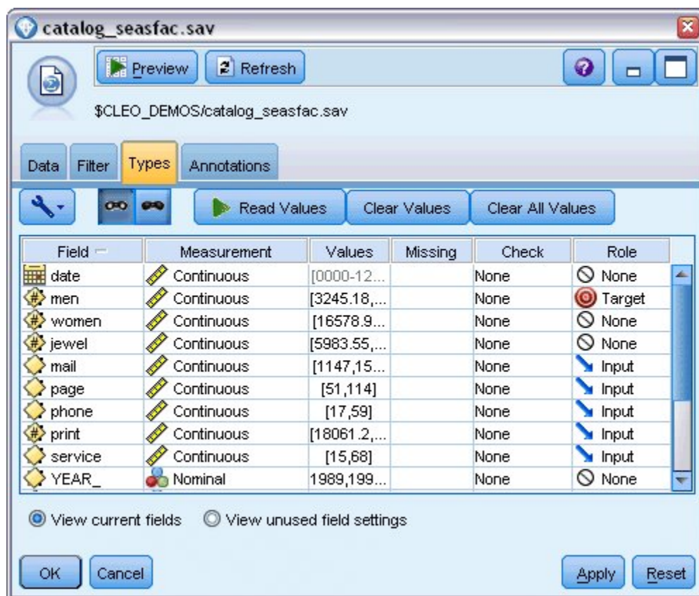
Figura 212. Configuración de los campos predictores
