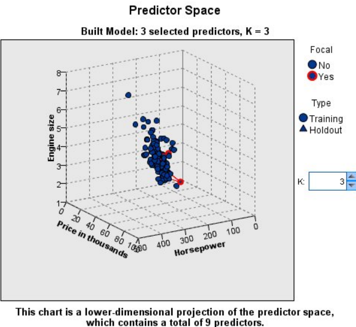
Figura 392. Gráfico Espacio predictor
