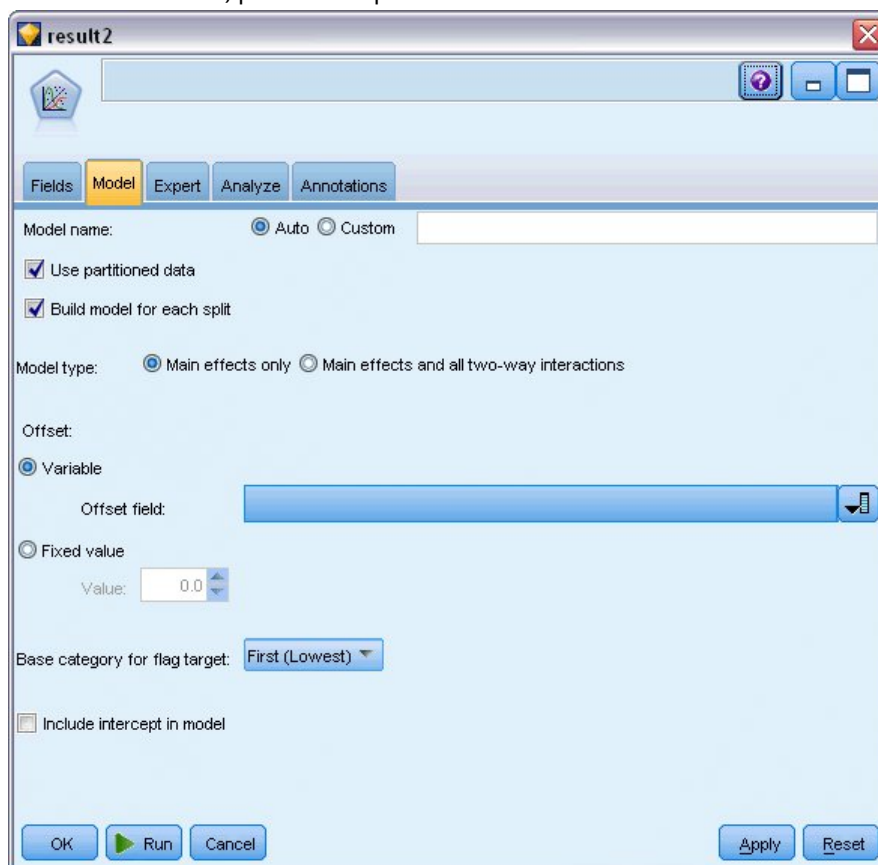
Figura 299. Selección de opciones del modelo
