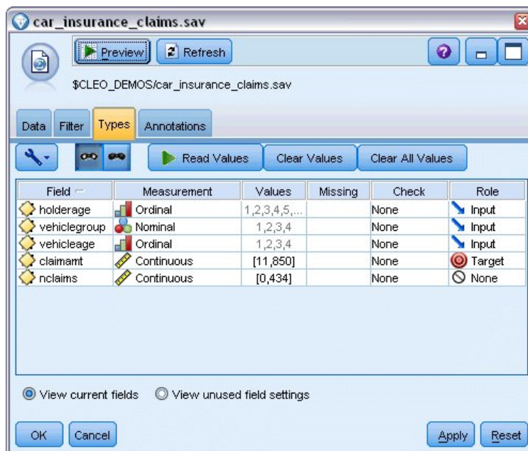
Figura 323. Definición del rol de campos
