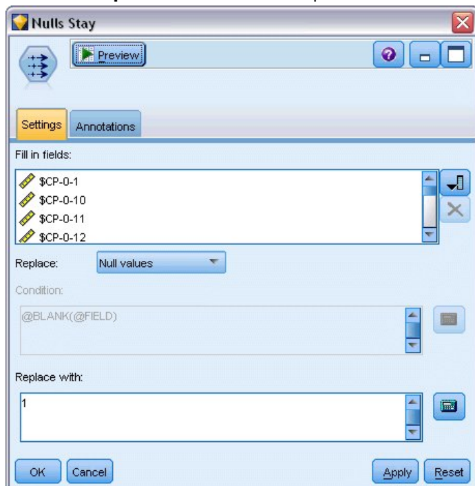
Figura 361. Nodo Rellenar: pestaña Configuración
