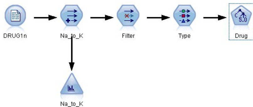
Figura 95. Adición de un nodo C5.0
