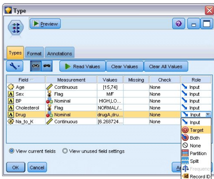
Figura 94. Edición del nodo Tipo
