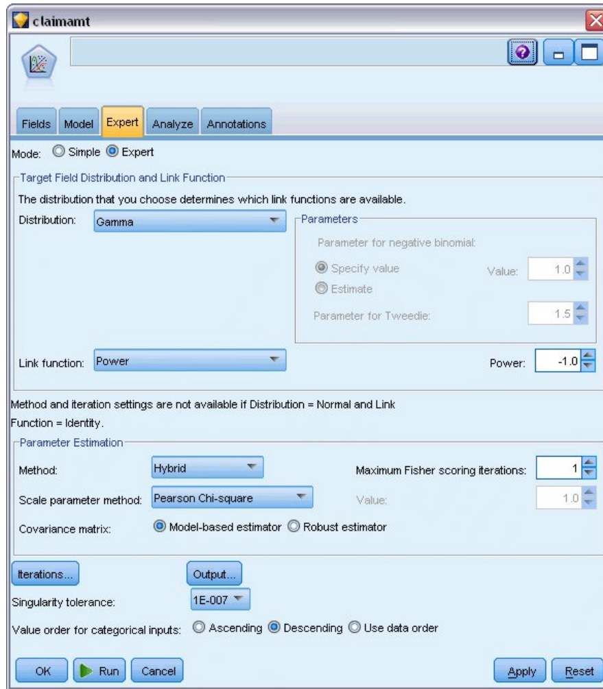
Figura 325. Selección de opciones de experto
