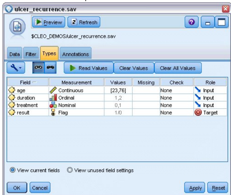
Figura 282. Definición del rol de campos
