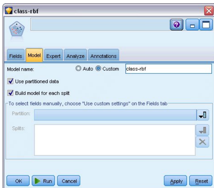
Figura 330. Configuración de la pestaña Modelo
