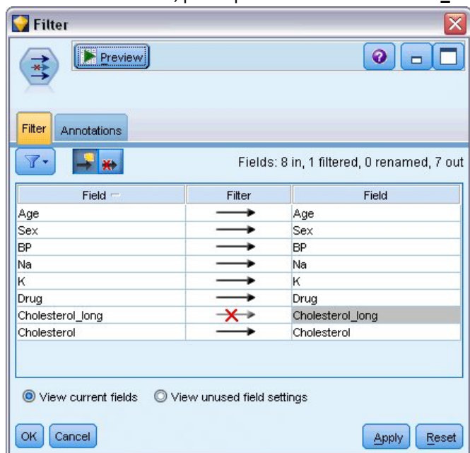
Figura 112. Filtrado del campo "Colesterol_alto" de los datos
