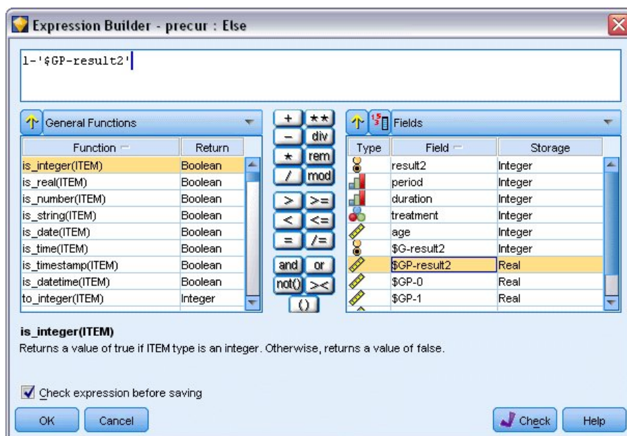
Figura 307. Nodo Derivar: Generador de expresiones de la expresión En caso contrario
