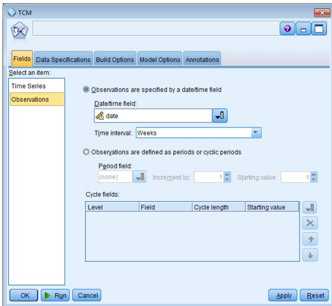
Figura 399. Modelado causal temporal, observaciones
