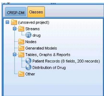
Figura 9. Vista Clases
