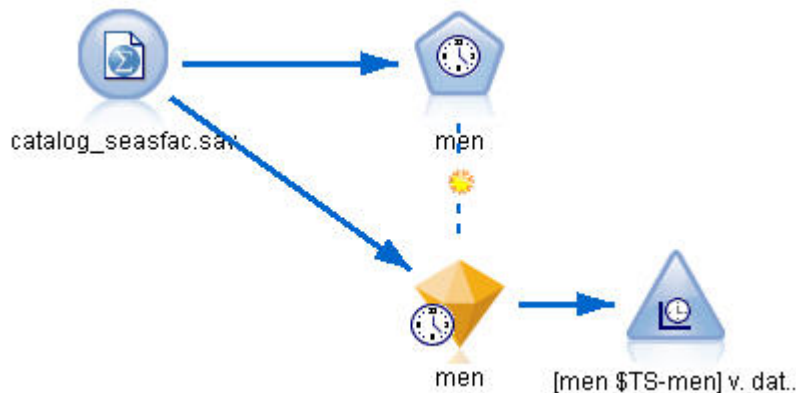
Figura 199. Previsión de ventas por catálogo
