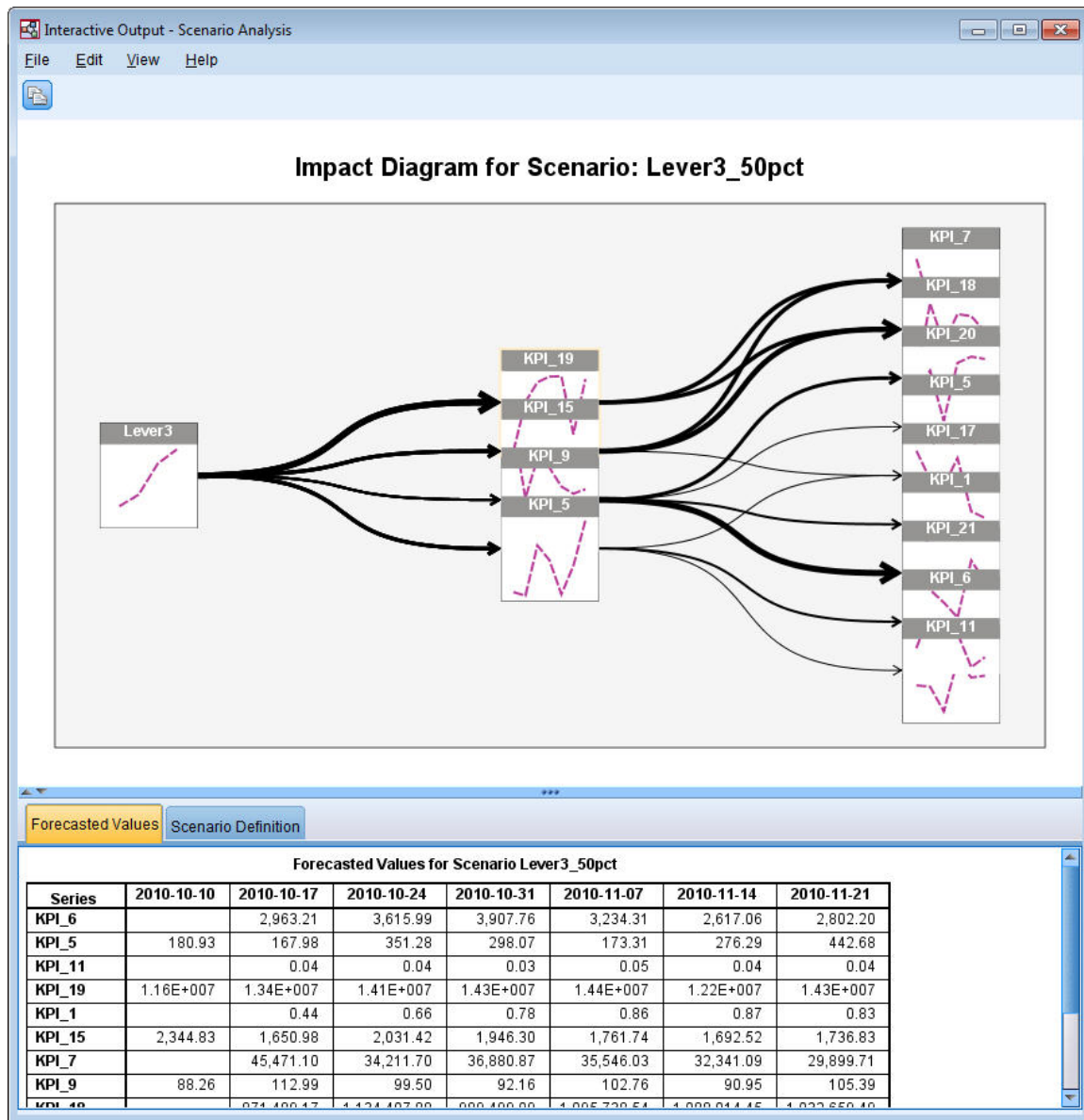
Figura 412. Diagrama de impacto para escenario: Lever3_50pct
