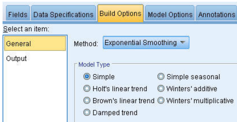
Figura 203. Especificación de suavizado exponencial
