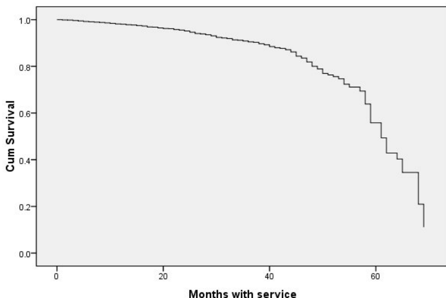
Figura 351. Curva de supervivencia de cliente "promedio"
