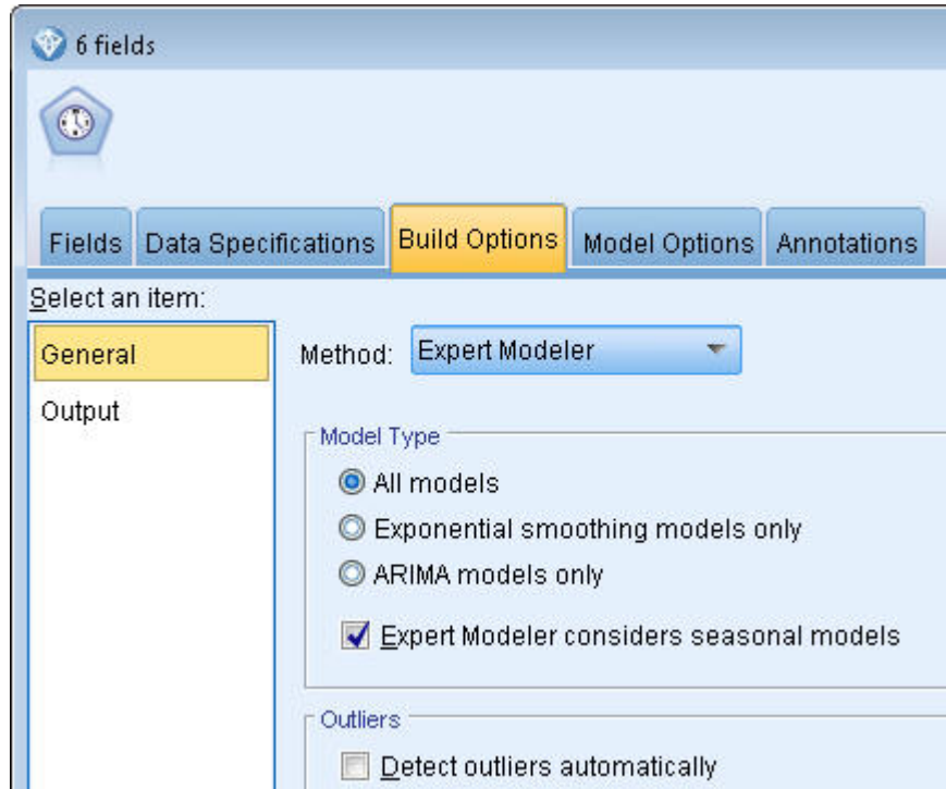
Figura 182. Selección del modelizador experto para series temporales
