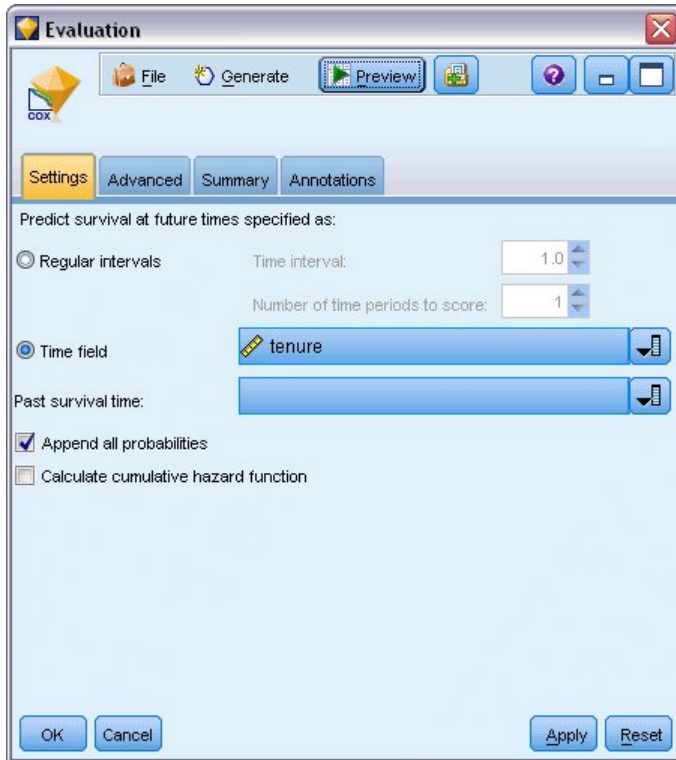
Figura 353. Nugget de Cox: pestaña Configuración
