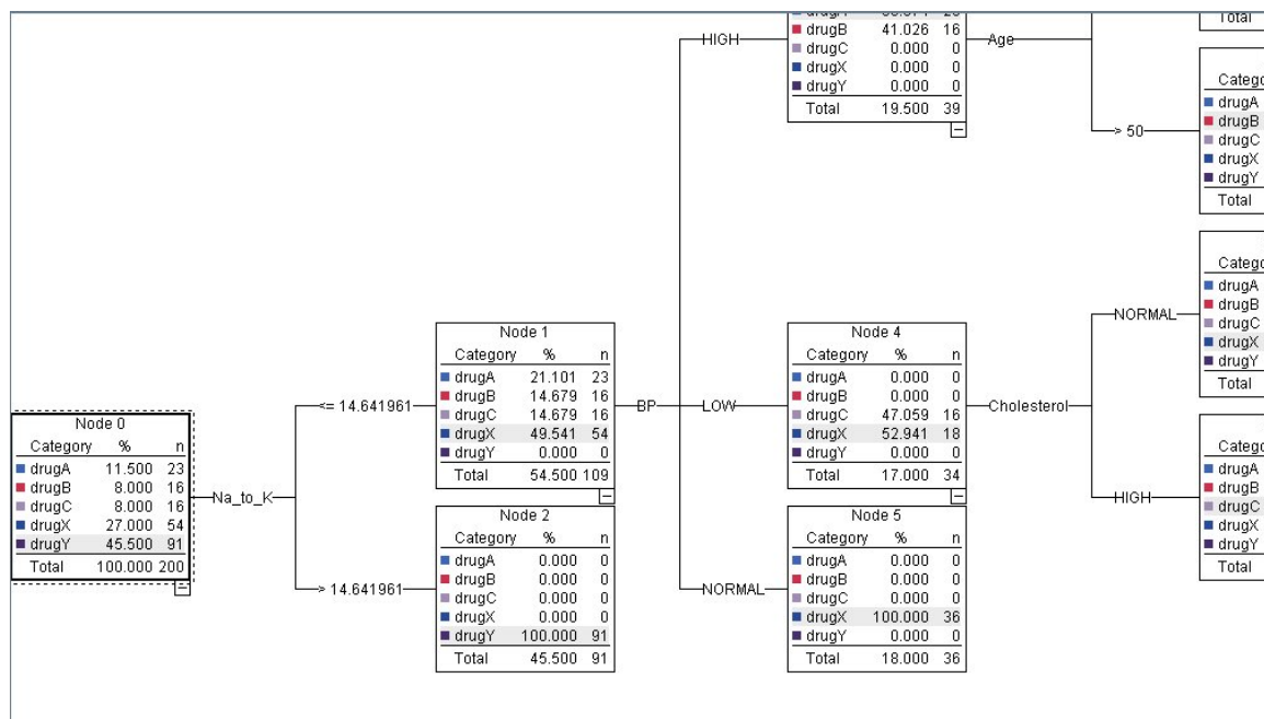
Figura 99. Árbol de decisión en formato gráfico
